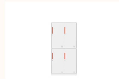
ME 四门更衣 H1850*W900*D500
